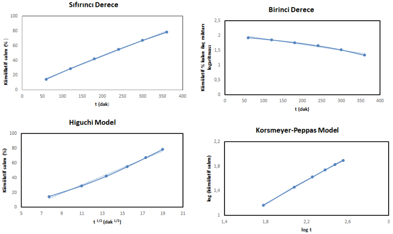
Şekil 5. PVA/HPMC membranlarına ait ilaç salım profilleri
