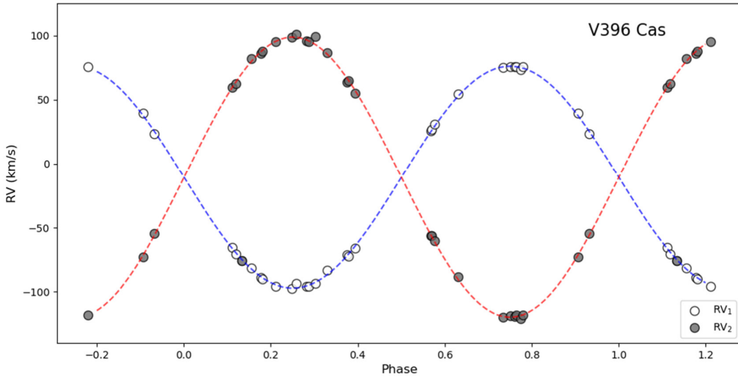
Şekil 2. V396 Cas'ın Lacy ve ark (2004)'nın RV eğrisi ile bu çalışmada WD yöntemi elde edilen kuramsal eğrinin uyumu görülmektedir. İçi boş daireler birinci bileşene ait, içi dolu daireler ikinci bileşene ait verilerdir.
