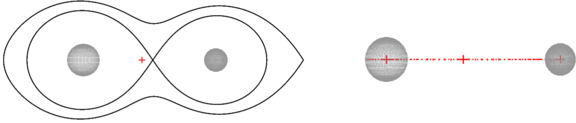
Şekil 5. V396 Cas'ın ışık eğrisi çözümünden elde edilen parametre değerlerine göre Roche geometrisi.
