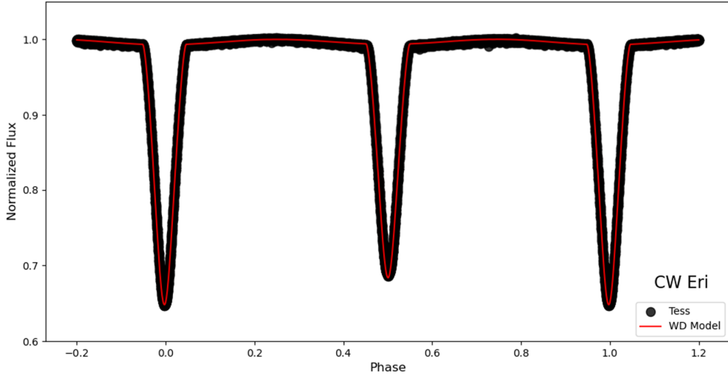
Şekil 3. CW Eri'nin TESS verilerinden elde edilen gözlemsel eğrinin, WD yöntemi ile elde edilen kuramsal eğri ile karşılaştırılması görülmektedir.
