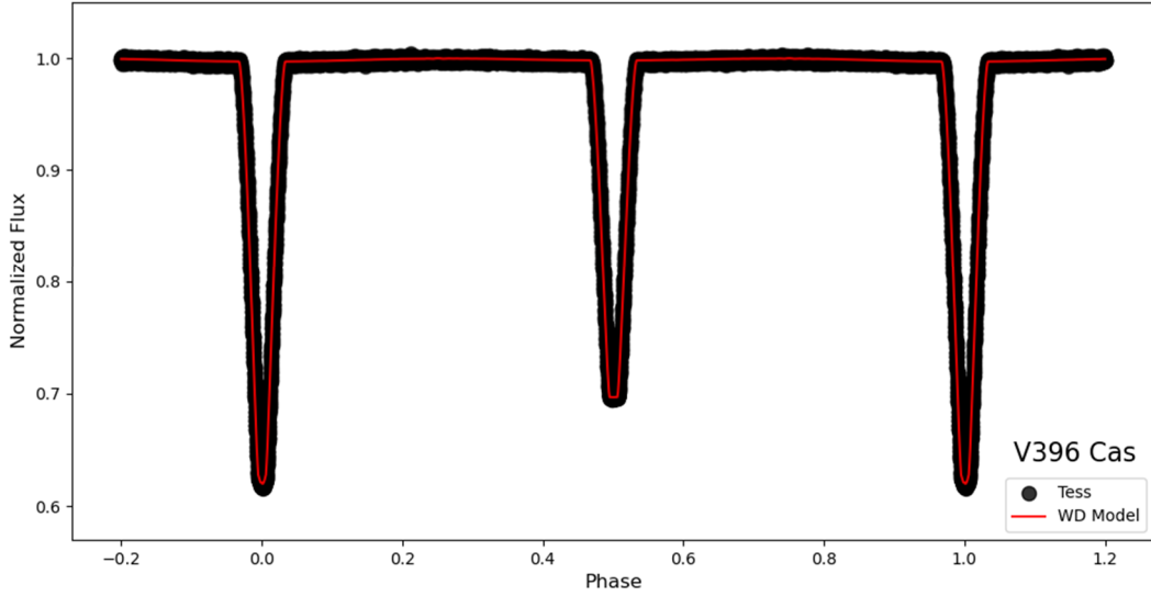
Şekil 1. V396 Cas'ın TESS verilerinden elde edilen gözlemsel eğrinin, WD yöntemi ile elde edilen kuramsal eğrinin karşılaştırılması görülmektedir.
