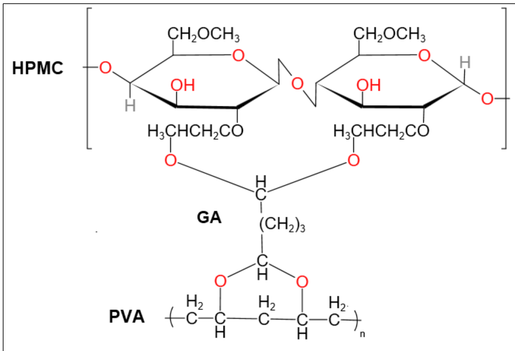
Şekil 1. PVA ve HPMC'nin GA ile çapraz bağlanma mekanizması [11].
