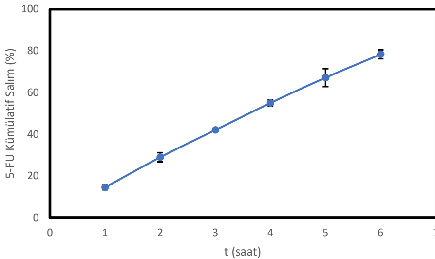
Şekil 4. 5-FU’in kümülatif salımı (5-FU: 200 mg; pH: 7,4; T= (37 ± 1) °C)
