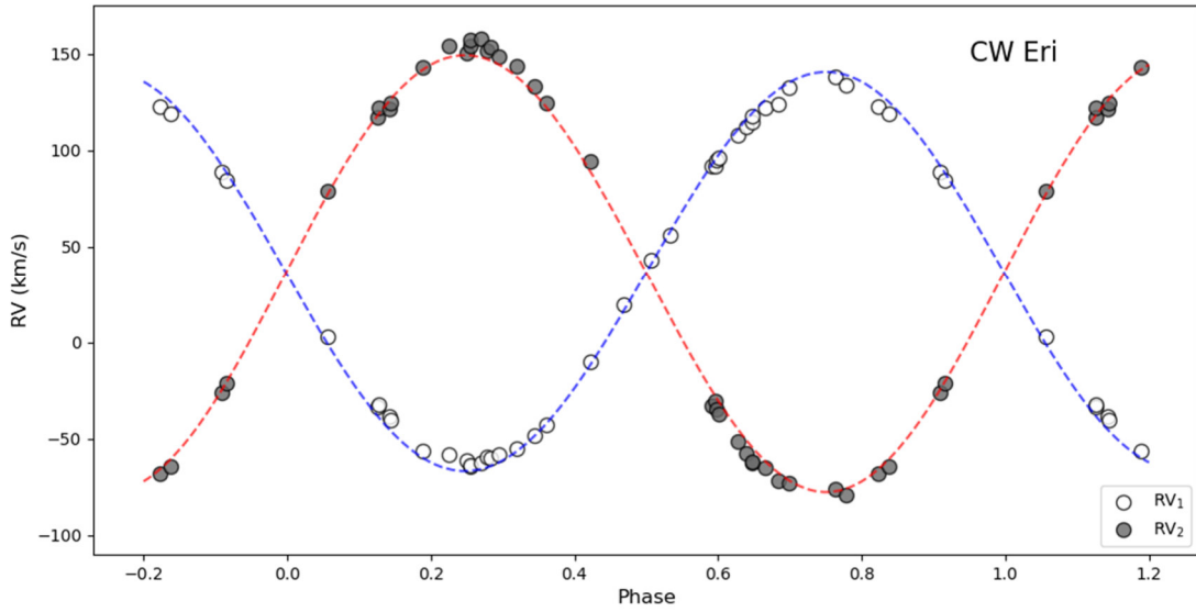
Şekil 4. CW Eri'nin Popper (1983) RV eğrisi ile bu çalışmada WD yöntemi elde edilen kuramsal eğrinin uyumu görülmektedir. İçi boş daireler birinci bileşene ait, içi dolu daireler ikinci bileşene ait verilerdir.
