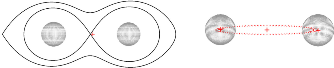
Şekil 6. CW Eri'nin ışık eğrisi çözümünden elde edilen parametre değerlerine göre Roche geometrisi.
