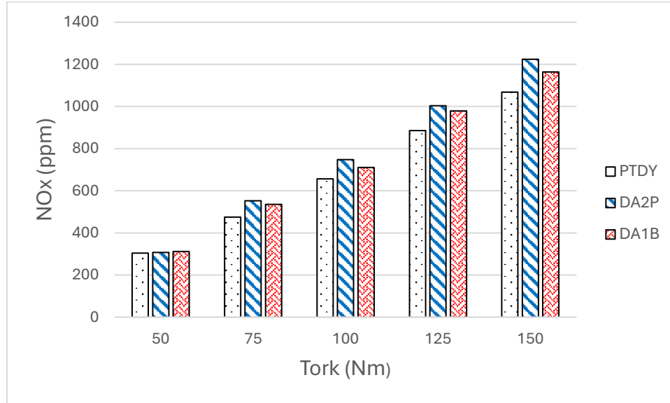
Şekil 4. \text{NO}_x Emisyonları
