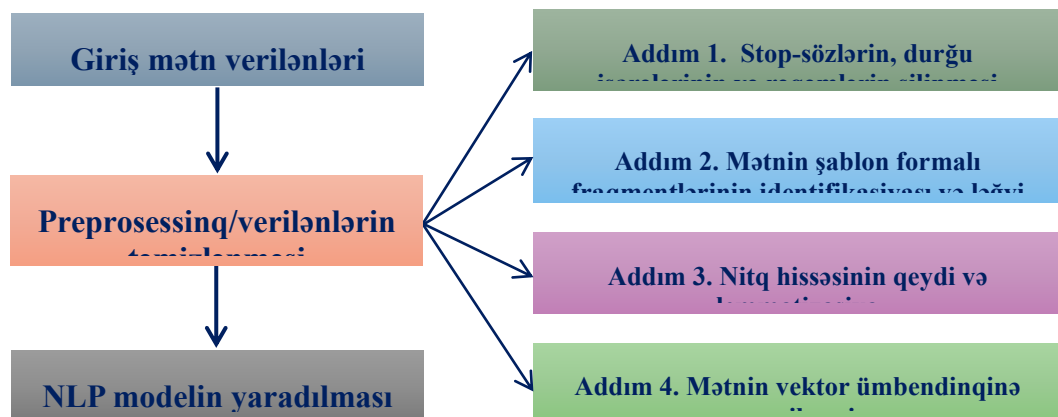
Səkil 2. Pipeline konveyeri vasitəsi ilə verilənlərin ilkin emalı sxemi (müəllif).
